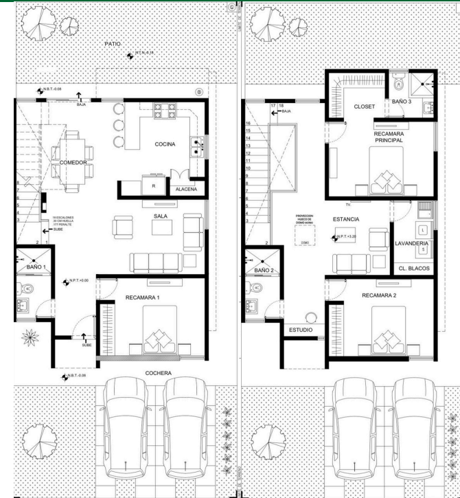
PLANTA BAJA PLANTA ALTA
